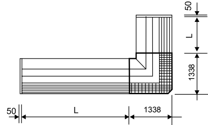
2) Geschlossener Winkel 90°
