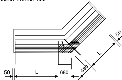
4) Geschlossener Winkel 135°
