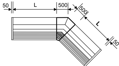
3) Offener Winkel 135°
