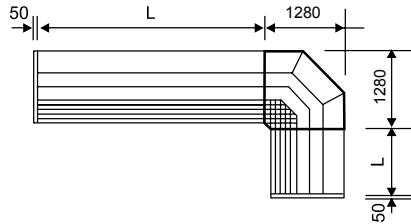
1) Offener Winkel 90°
